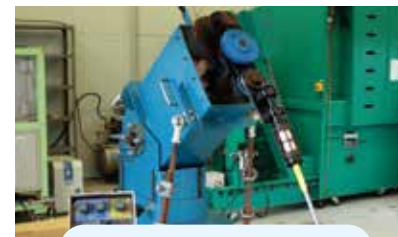
弾道実験のためのスイングロボット
